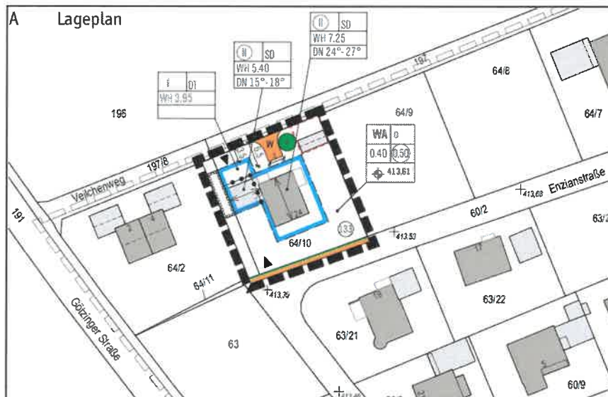
Lageplan
